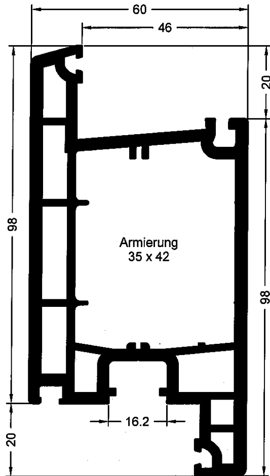
Art. 541130 01 Art. 541350 kaschiert Haustürflügel Z TD
