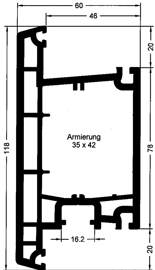
Art. 541150 01 Art. 541340 kaschiert Haustürflügel T TD
