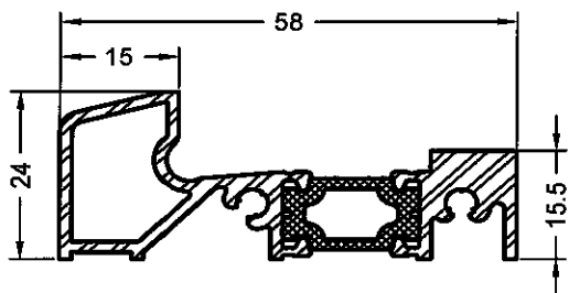
Art. 260000 natur eloxiert Aluminium Bodenschwelle Altbau TD
