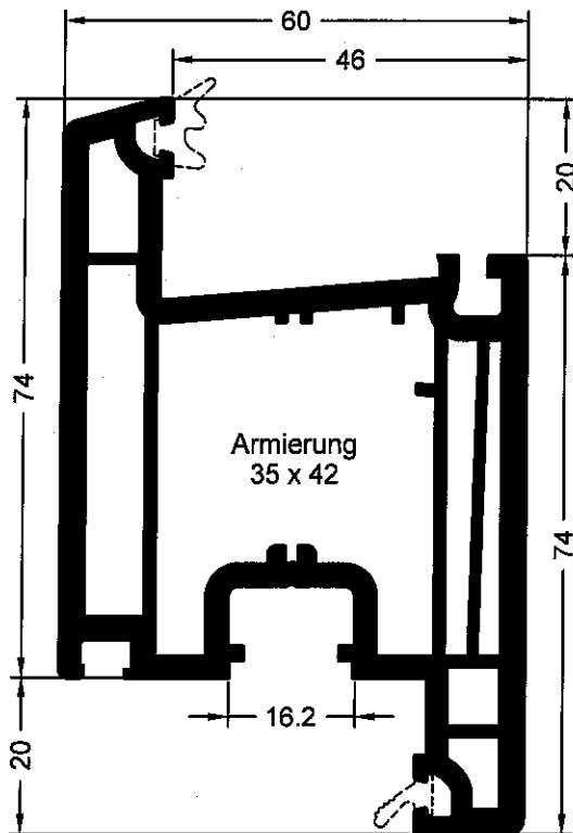
Art. 554081/554085 01, 15 Art. 564081/564085 kaschiert Flügel Z 74 TD/Flügel Z 74 TD mit verschweißbaren Dichtungen
