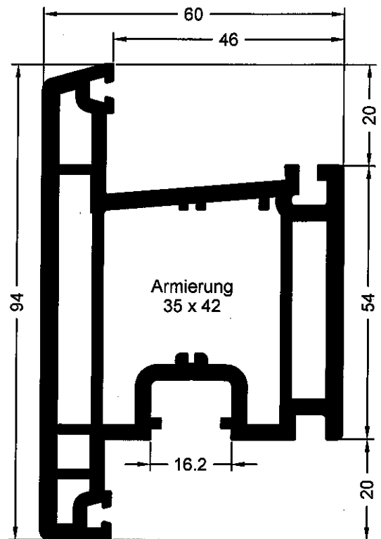
Art. 541170 01 Art. 541330 kaschiert Flügel T 94 TD
